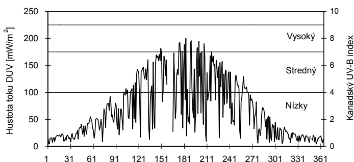
Obr. 3.4 Ročný chod poludňajších hodnôt DUV (Diffey) žiarenia – Gánovce 2003
