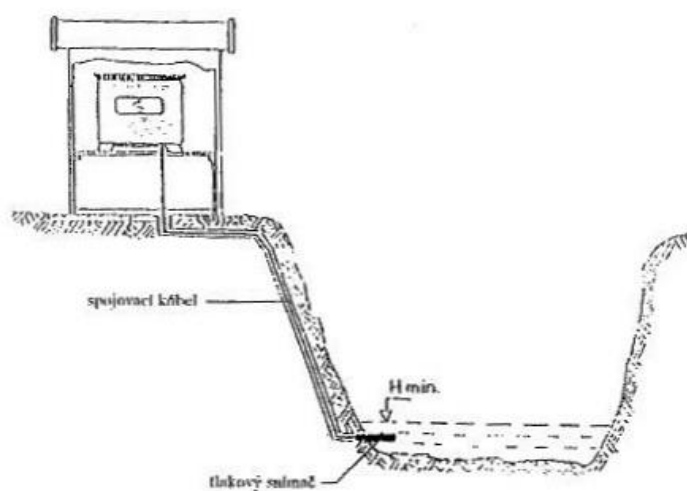
REGISTRAČNÉ STANICE S TLAKOVÝM SNÍMAČOM (odporúčaná vzor)
