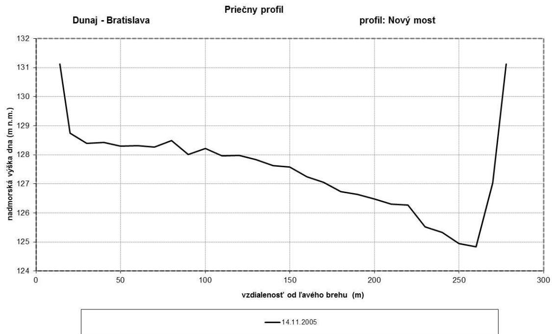
Obr. 4 Priechny profil – Dunaj v Bratislave, pod Novým mostom
