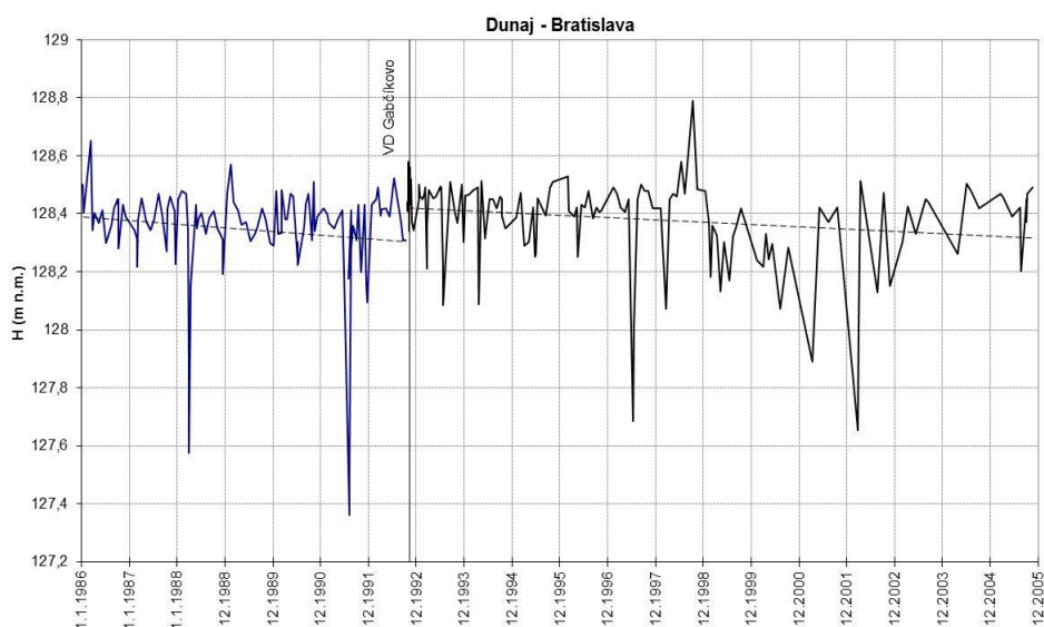
Obr. 8 Zmeny úrovně dna v zvislici 80 m od ľavého brehu
