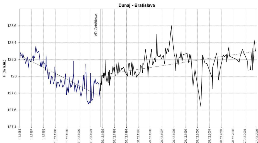
Obr. 7 Zmeny úrovně dna v zvislici 50 m od ľavého brehu
