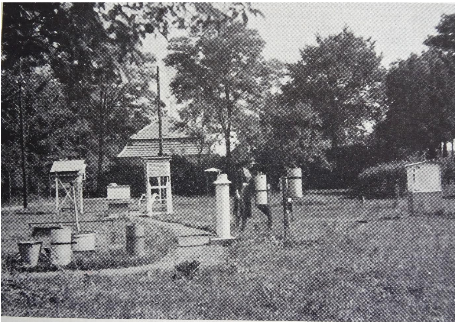
Obr. 3. Celkový pohľad na umiestenie meteorologických búdok, v popredí zrážkomerv.
